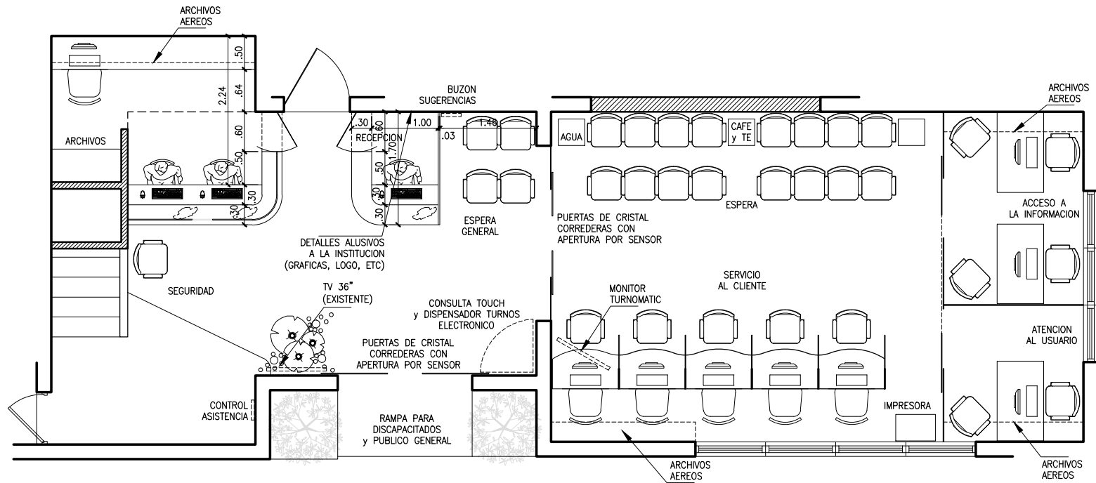
Planta Amueblada Esc.: 1/50
